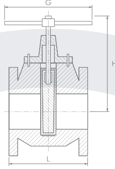
ÖLÇÜLER / DIMENSIONS
